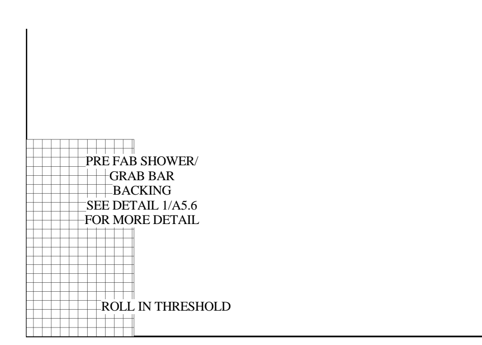
4 M/ SHOWER N. WALL 3/8" = 1'-0"
